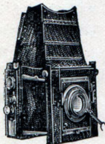
ベンチン疊込レフ
