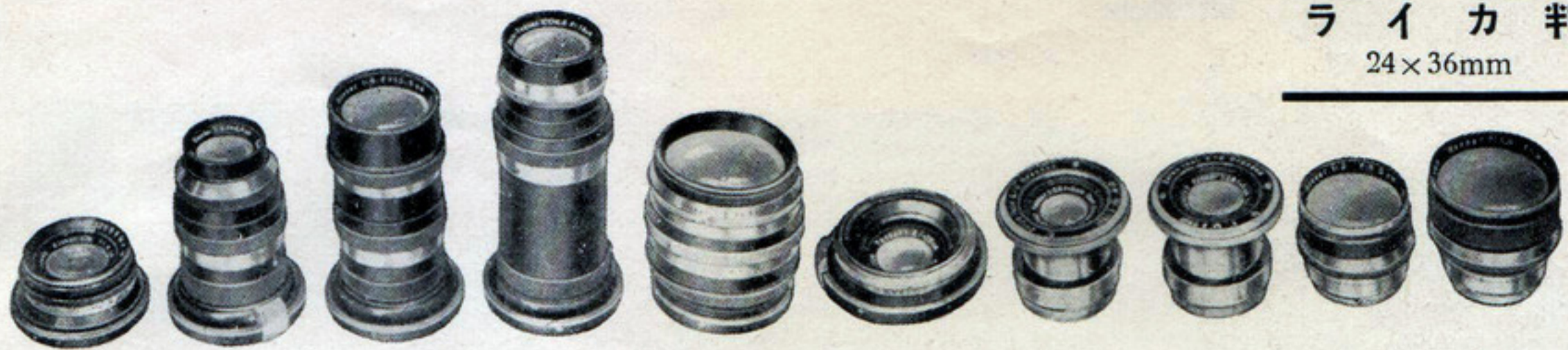
ピオター F2/4cm トリオター F4/8.5cm ゾナー F4/13.5cm テレテツサー-K F6.3/18cm ゾナー F2/8.5cm テツサー F8/2.8cm テツサー F3.5/5cm テツサー F2.8/5cm ゾナー F2/5cm ゾナー F1.5/5cm
