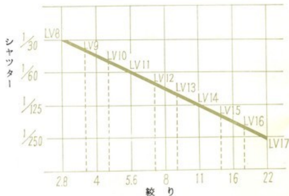
キヤノンデミプログラムシャッター変化図
