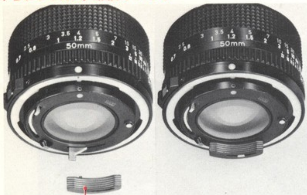
絞りレバーストッパー
